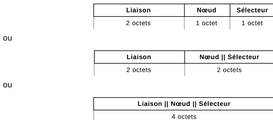
Figure 4 – Variantes de structures d'adresse de DL
