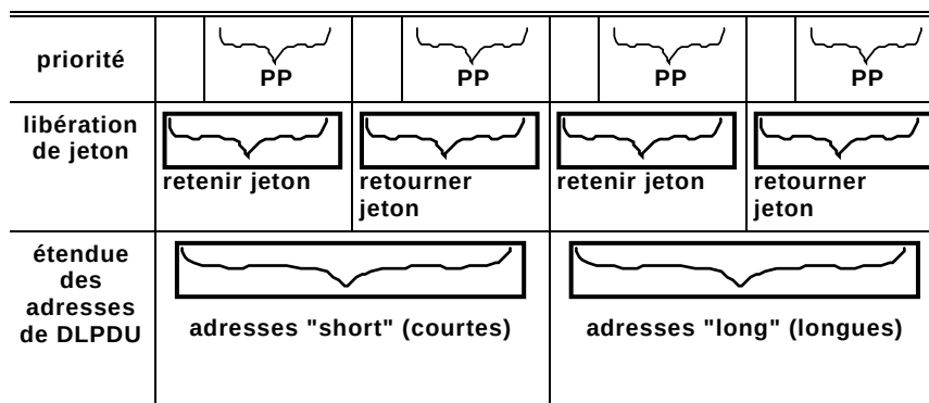
Figure C.1 – Structure grossière des points de code de FC
