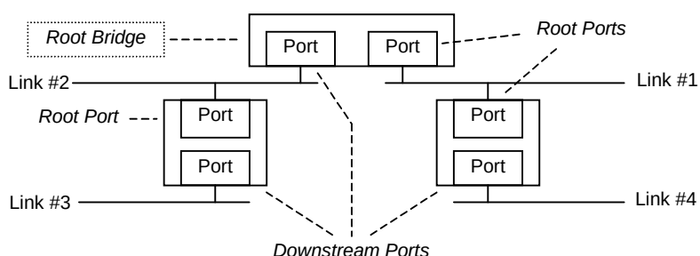
Figure 14 – Topologie de réseau ponté
